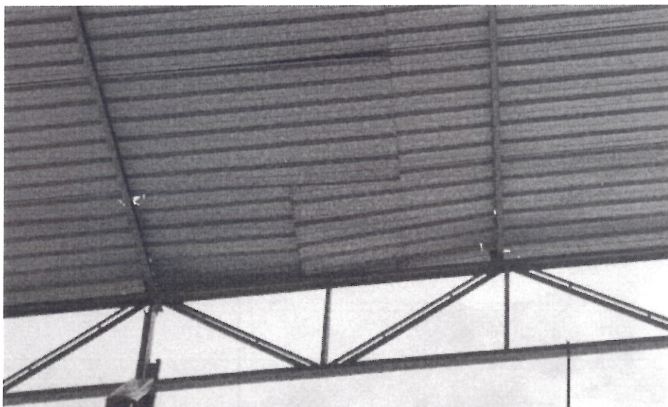
Imagem 04: Quadra Poliesportiva do Distrito do Campestrinho com telhas da cobertura com extremidades soltas. – Arquivo da Divisão de Planejamento Urbano.
