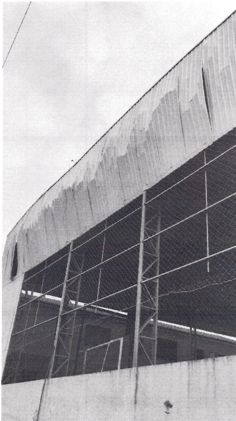
Imagem 01: Quadra Poliesportiva do Distrito do Campestrinho com a presença de danos em seu fechamento lateral. – Arquivo da Divisão de Planejamento Urbano.
