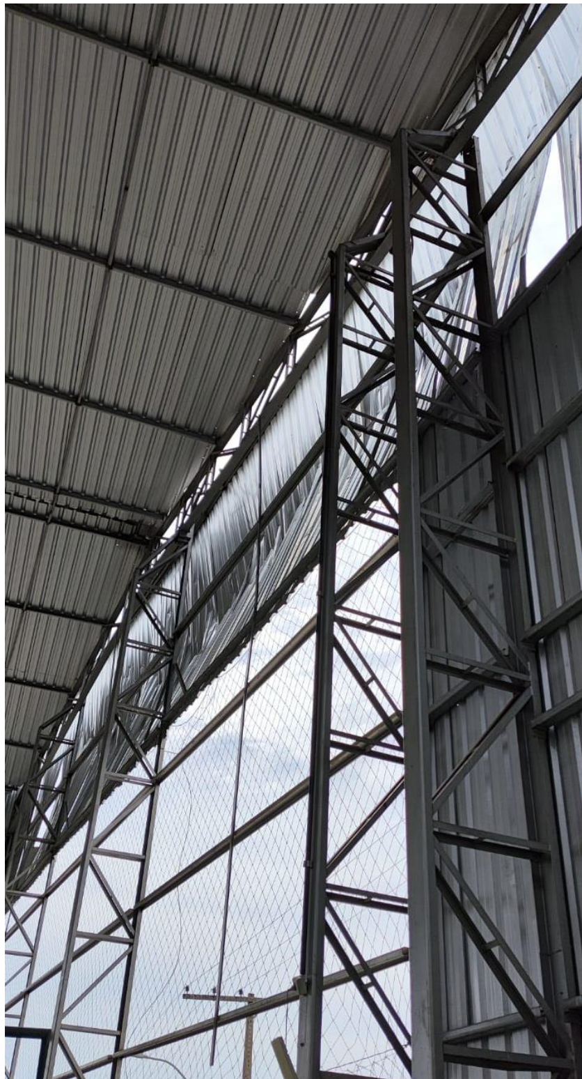
Imagem 03: Quadra Poliesportiva do Distrito do Campestrinho com a presença de danos em seu fechamento lateral. – Arquivo da Divisão de Planejamento Urbano.
