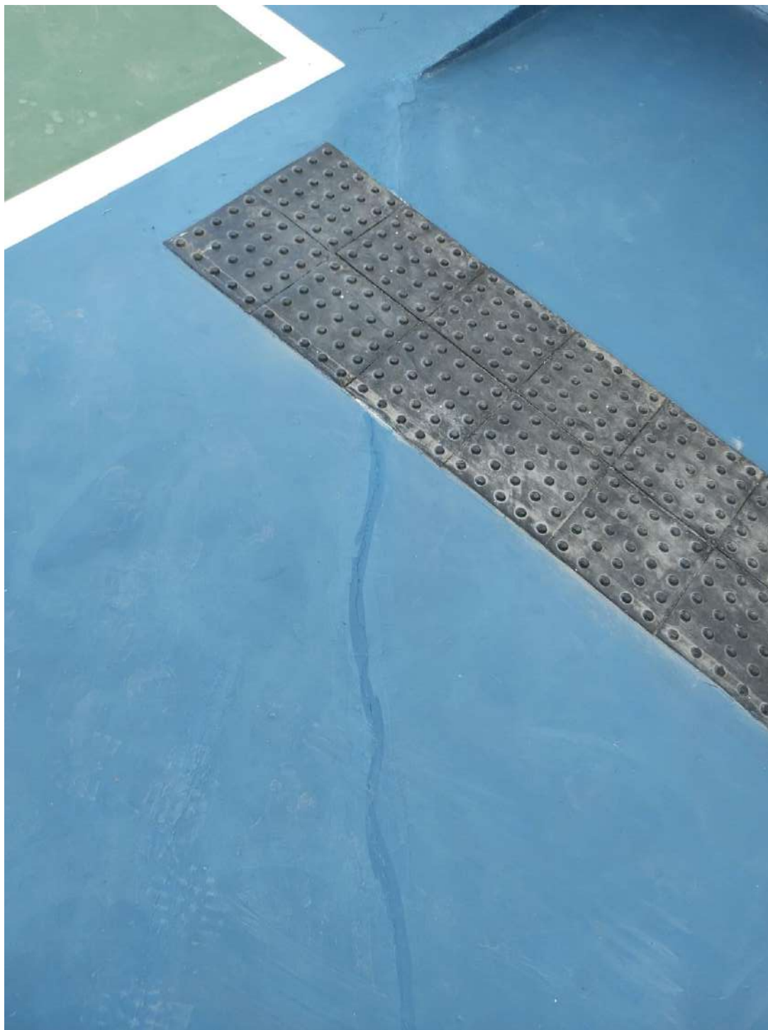
Imagem 33: Trincas no piso da quadra poliesportiva, na obra de Construção de Quadra Poliesportiva do Distrito do Campestrinho. Arquivo da Divisão de Planejamento Urbano e Projetos.
